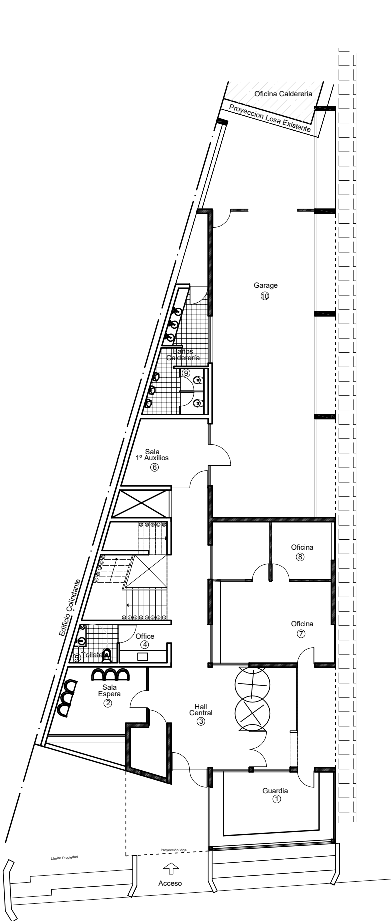
PLANTA NIVEL 0,25
